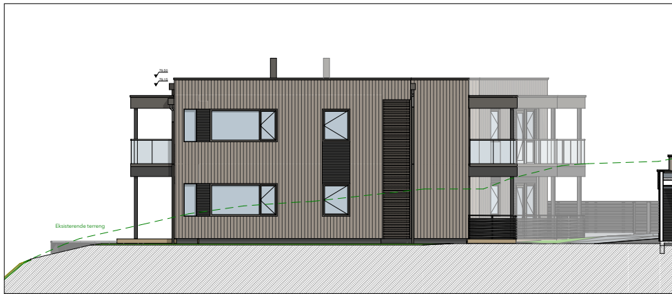
1:50 Fasade sør
