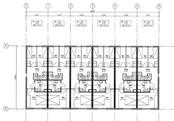
PLAN 2. etg. 7.888 m 2 x 297,3 m
