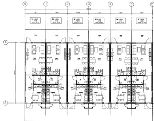
PLAN 1. etg. 7.888 m 2 x 297,3 m
