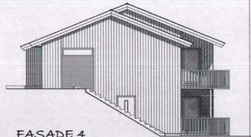
FASADE 4
