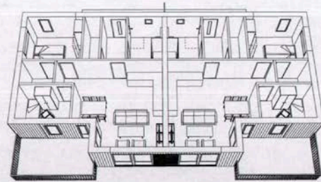
1. ETG.
