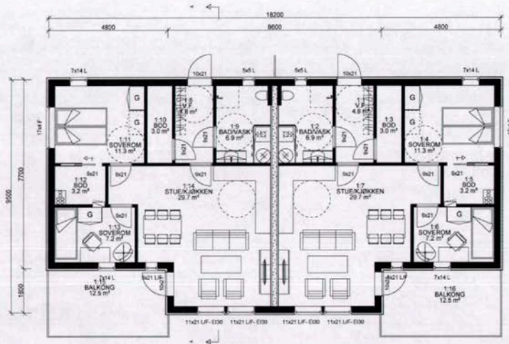
1. ETG.PLAN
