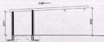
SNITT A-A
