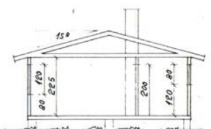
SNITT
