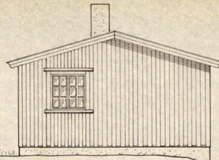
FASADE SYD.
