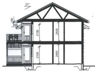
SNITT A - A
