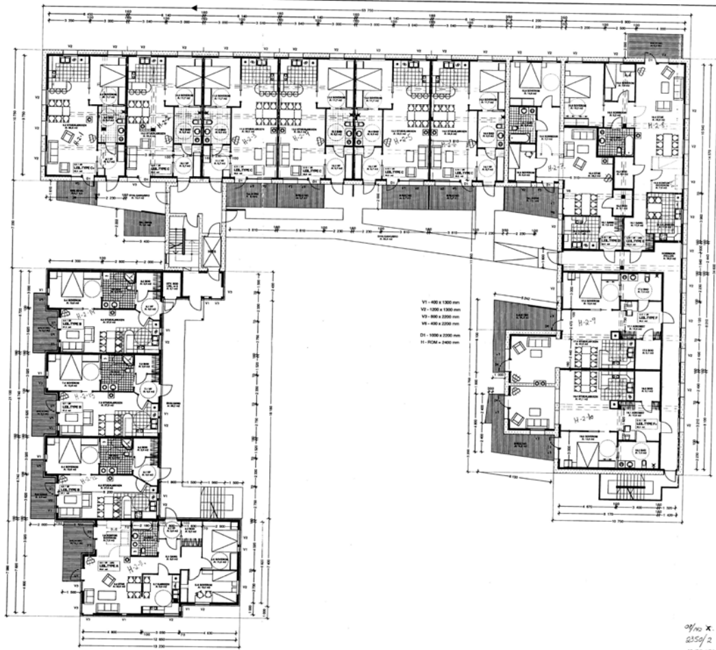
PLAN - 2 - ETG mál 1:100
