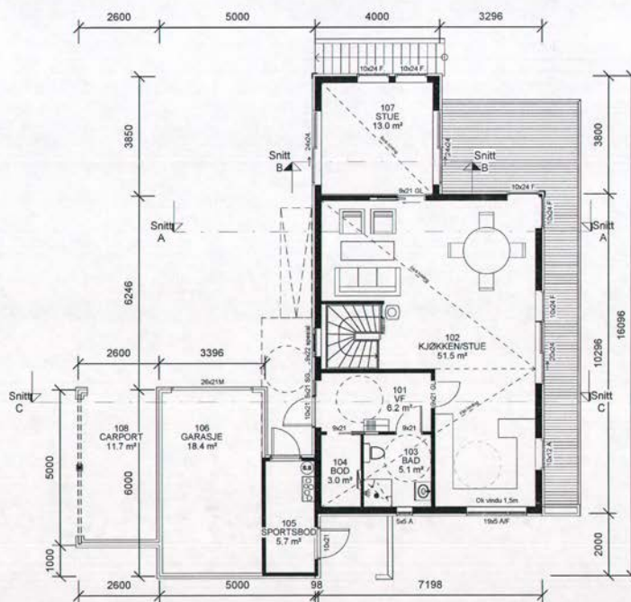
1. ETASJE
