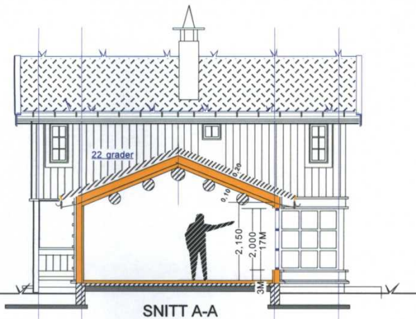
SNITT A-A
