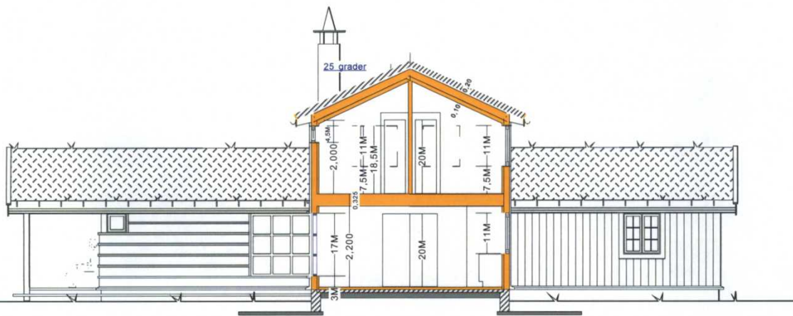
SNITT B-B
