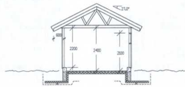
SNITT A-A
