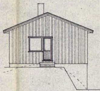
Fasade mot öst.
