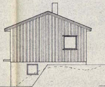
Fasade mot väst.
