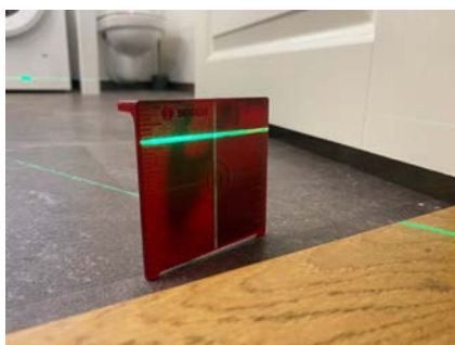
Måling av fall fra underkant terskel dør.
