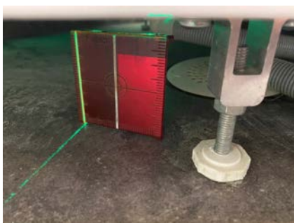
Måling av fall mot sluket.
