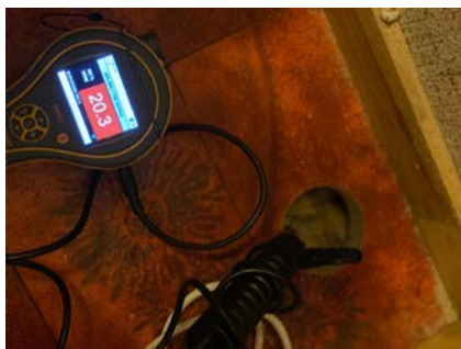
Fuktmåling foretatt med Protimeter MMS2 med pigger mot treverket i oppoforet gulv.
