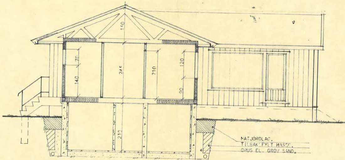
SNITT A-A
