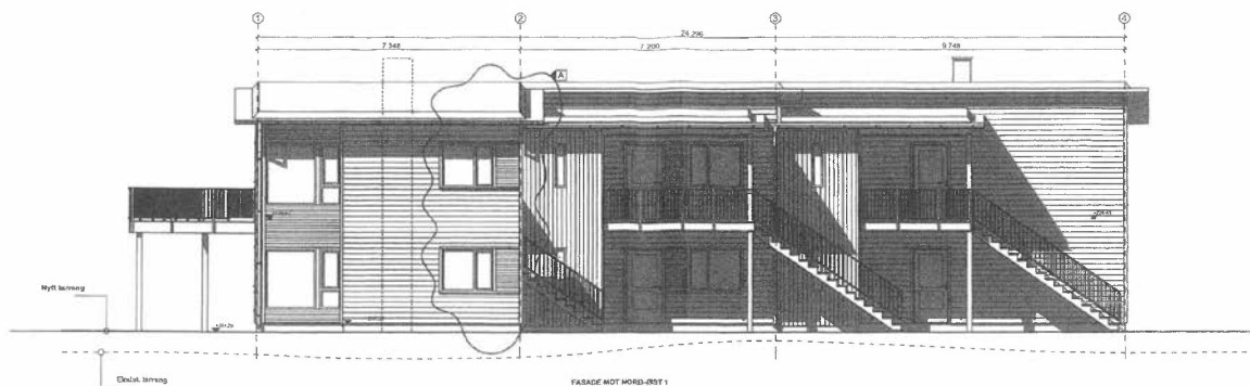
FASADE MOT NORD-ØST 1
