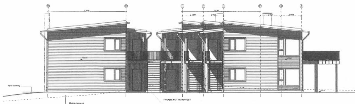
FASADE MOT NORD-VEST
