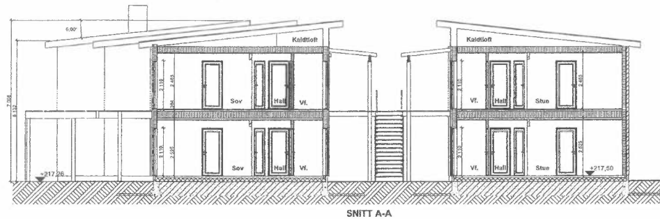
SNITT A-A
