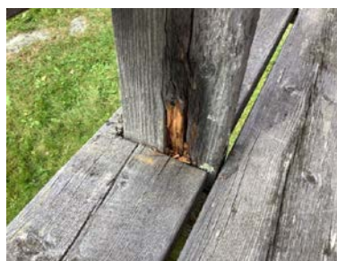
Råteskadet rekkverksstolpe.
