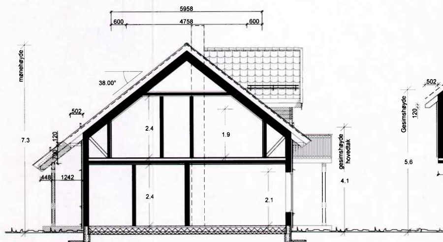
Snitt A-A
