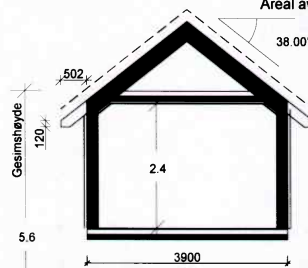
Snitt B-B
