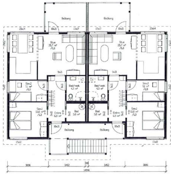
Plan 2. etasje
