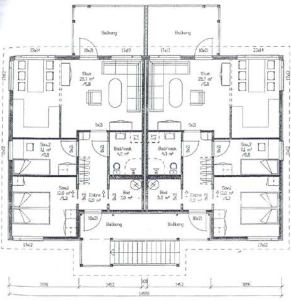
Plan 2. etasje
