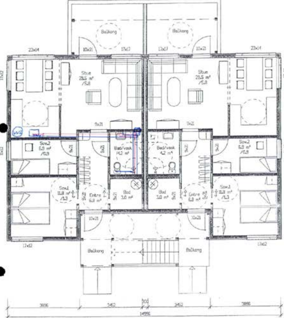
Plan 1. etasje
