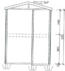
Snitt
