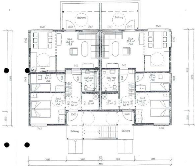
Plan 1. etasje
