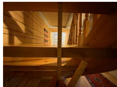
Åpning på 15cm mellom trinn.
