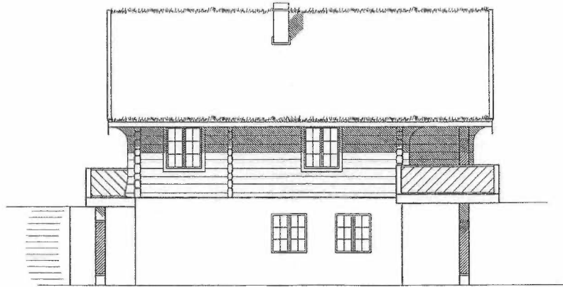
FASADE VEST
