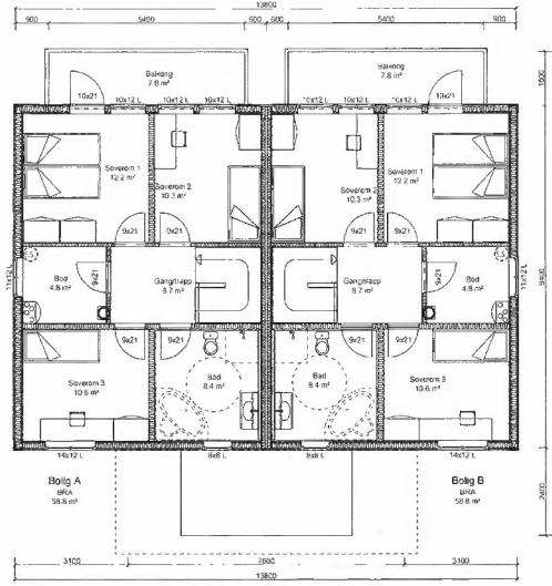
PLAN 2. ETASJE
