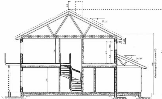
SNITT A - A
