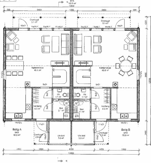
PLAN 1. ETASJE
