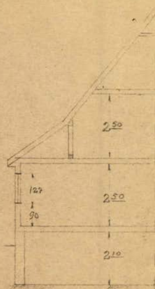
- SNITT -
