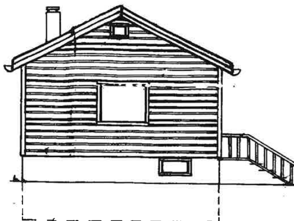
FASADE VEST
