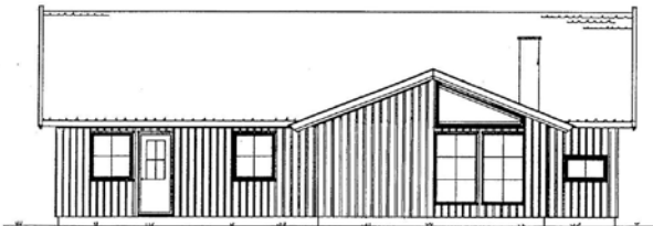
Fasade C mot
