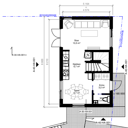
HUS A - 01 1:100
