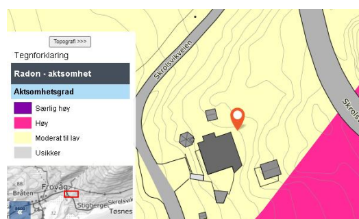
Radon aktsomhetsnivå.
