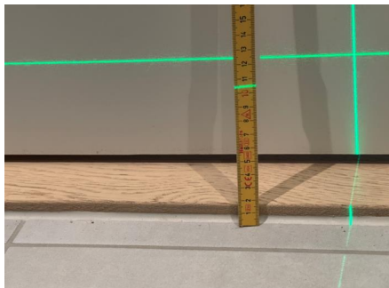
Fallforhold ca. 105 mm overkant gulv ved terskel
