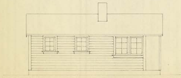
FASADER MÅL 1:100
