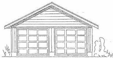
FASADER mål 1:100
