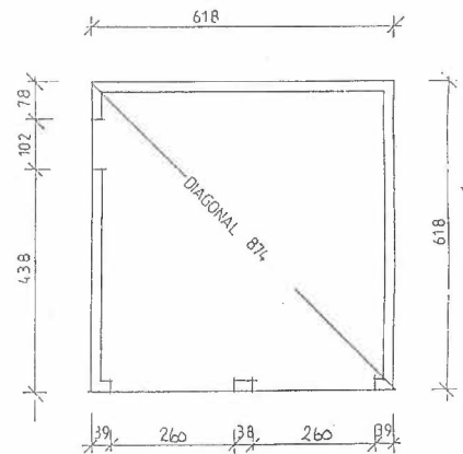
FUNDAMENT PLAN mål 1:100
