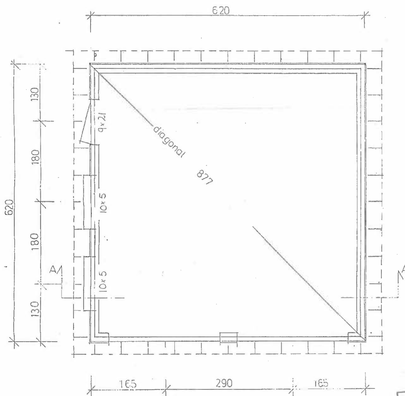
PLAN mål 1:50
