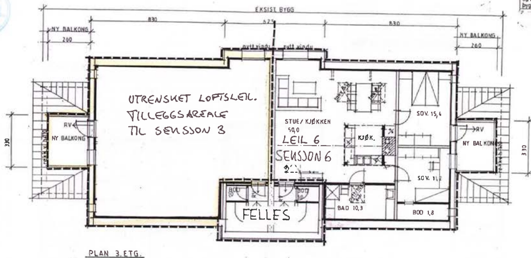
PLAN 3. ETG.
