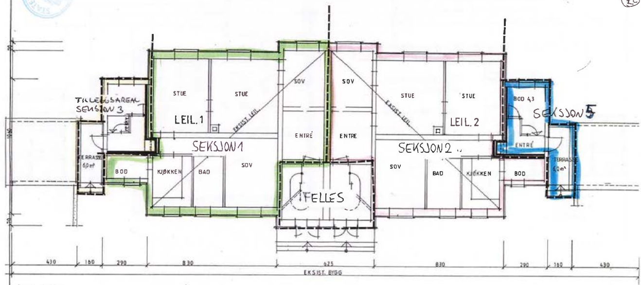
PLAN 1. ETG.
