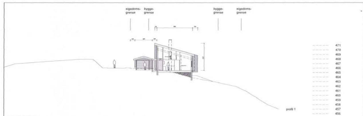
SNITT / PROFIL 1
