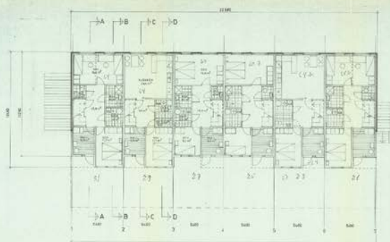
PLAN 1 ETO.
