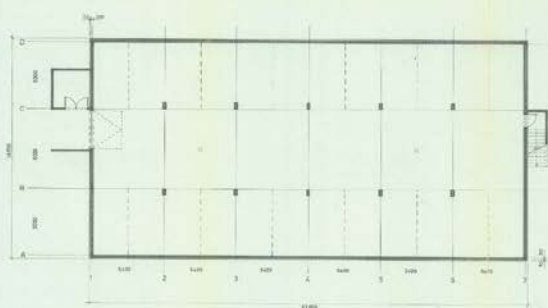
PLAN GARASJEKJELLER
