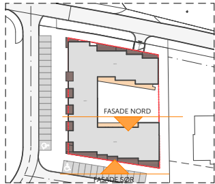
SITUASJONSKART 1:1000
