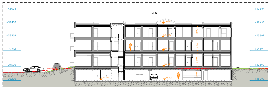
SNITT A-A 1:200
