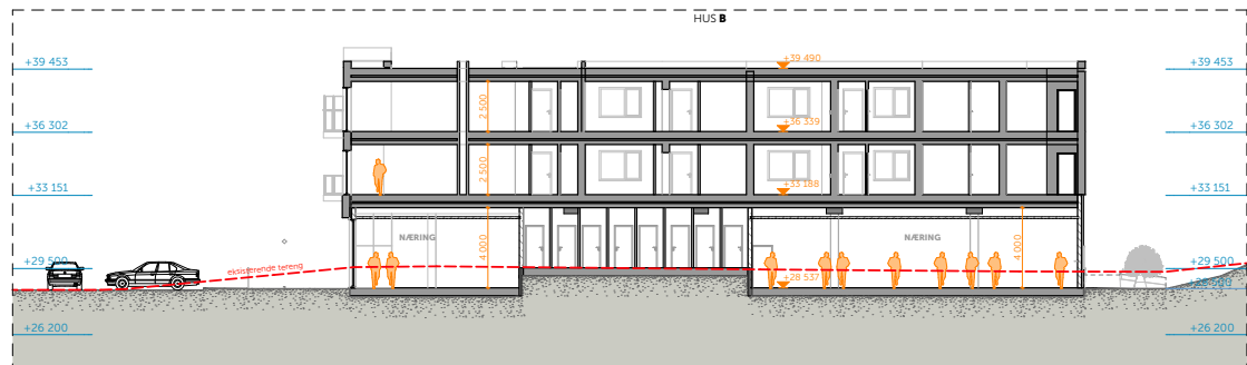
SNITT B-B 1:200
