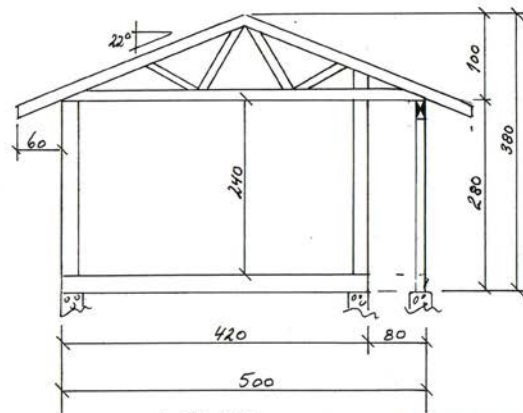
Snitt tilbygg
