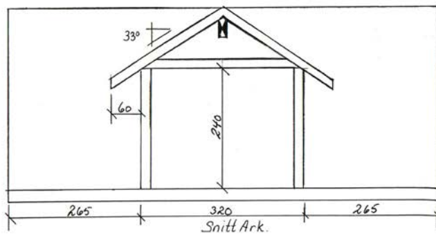
Snitt Ark.
