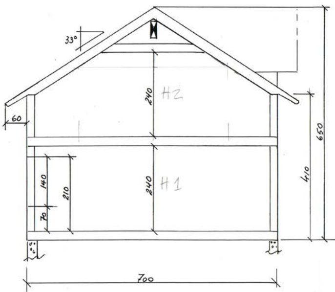
Snitt hovedbygg
