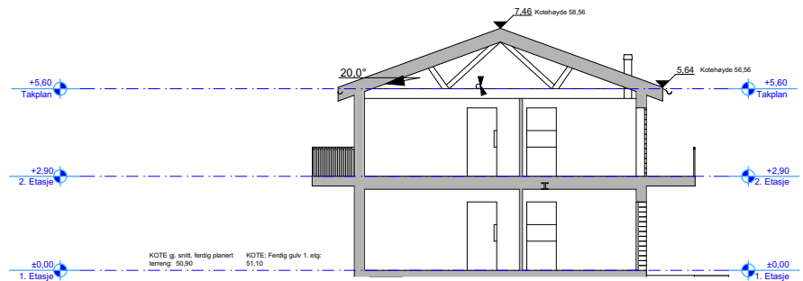
1:100 Snitt A
