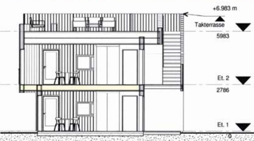
Snitt B 1 : 100
