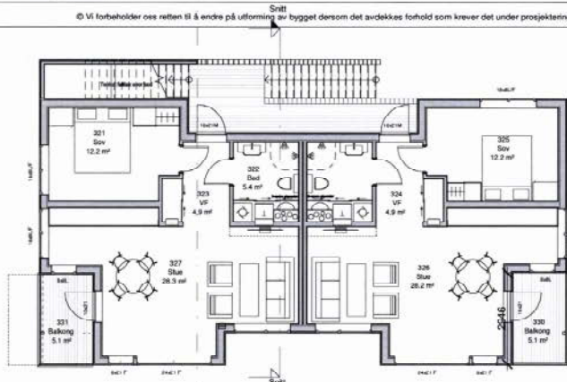
PLAN 2. ETG. 1 : 100
