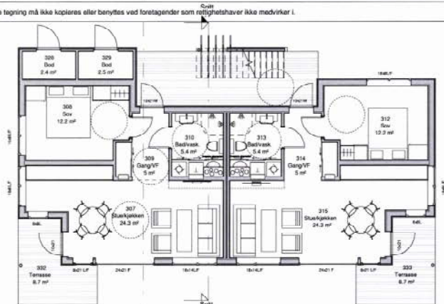
PLAN 1. ETG 1 : 100
