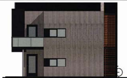
FASADE 2 1 : 100
