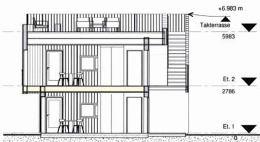
Snitt B 1 : 100
