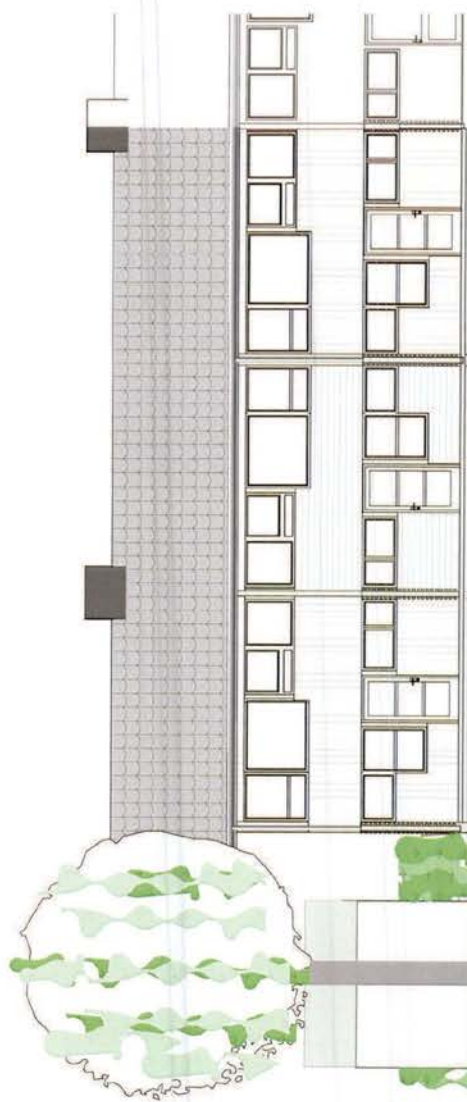
FASADE ØST Rekkehus B-vest; Nr 79-75
