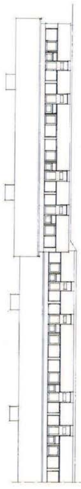
KOMPLEKSE/VEKST FOT. 13 OG 14. SNITT 13-14
