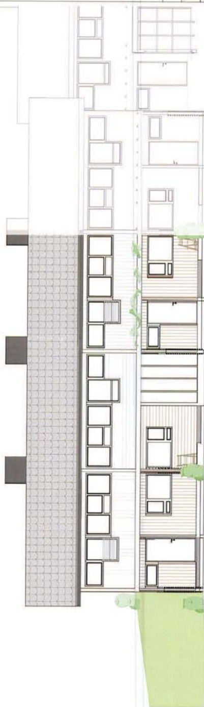
FASADE ØST Rekkehus C; Nr 35-29 Tak over inngangsparti legges i rammen.
