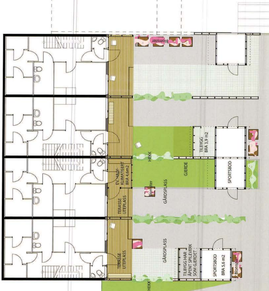
1.ETG. INNGANGSPLAN Rekkehus D, Nr 19-13
