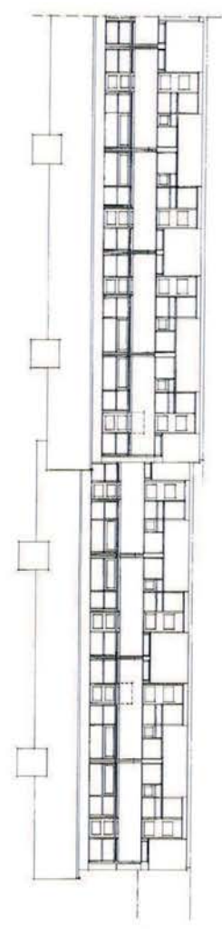
INDGANGSPARTI/VEKST FOT. 13 OG 14. SNITT 13-14
