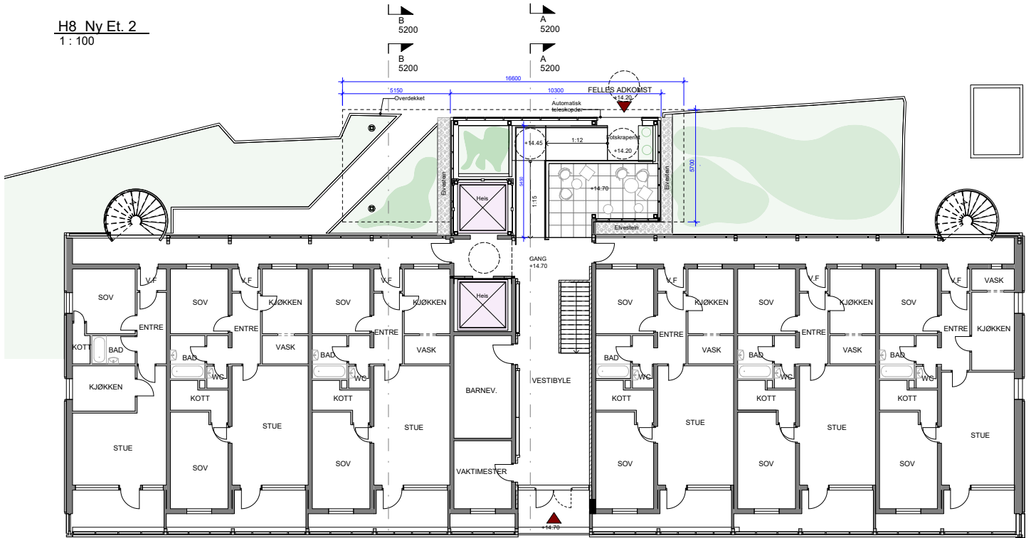
H8 Ny Et. 1 1:100
