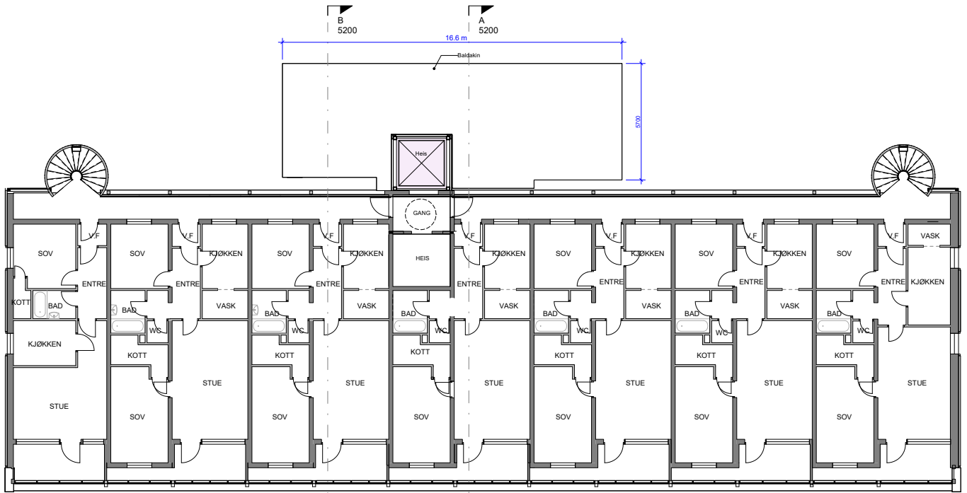
H8 Ny Et. 2 1:100
