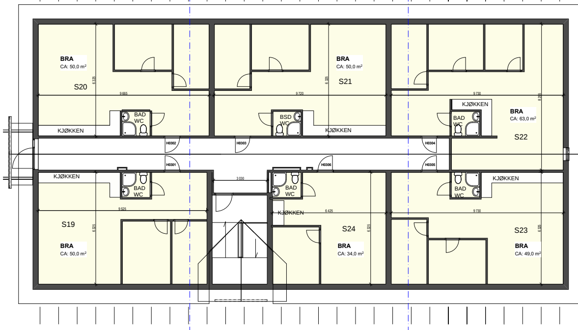
Takplan (1) 1:100
