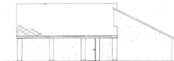
FASADE NØRØ-VEST
