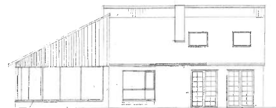
FASADE SØR-ØST
