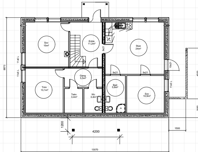
PLAN UNDERETASJE
