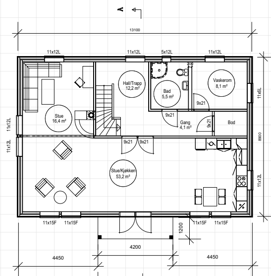
PLAN 1. ETASJE
