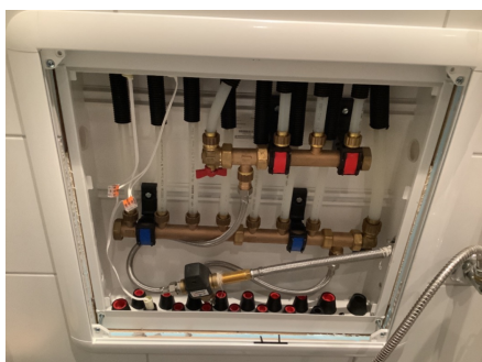
Vannfordelerskap i bad i 1. etg.
