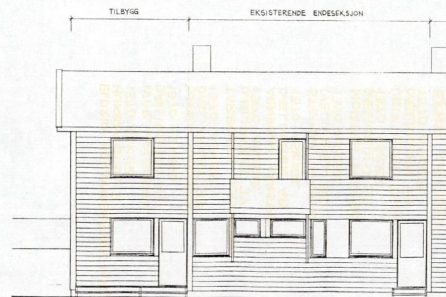
FASADE SYDØST
