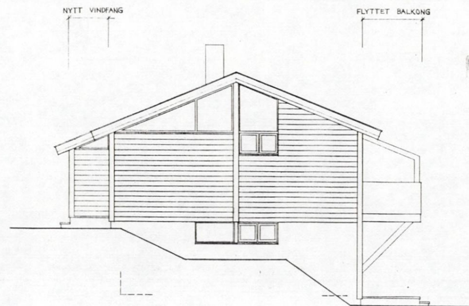
FASADE SYDVEST
