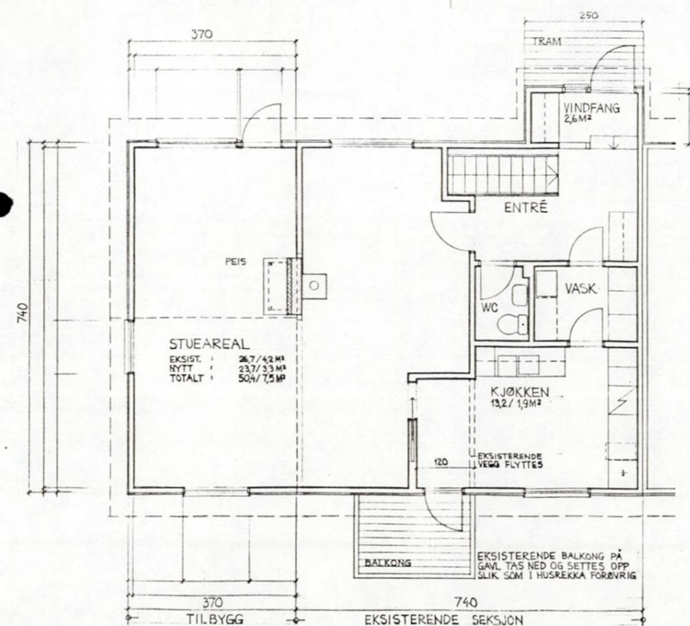
PLAN 1. ETASJE
