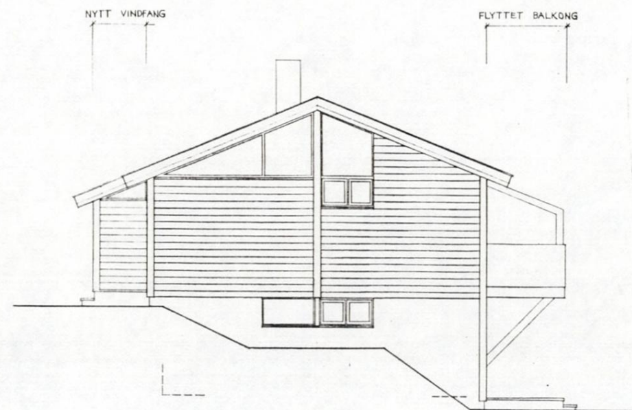
FASADE SYDVEST
