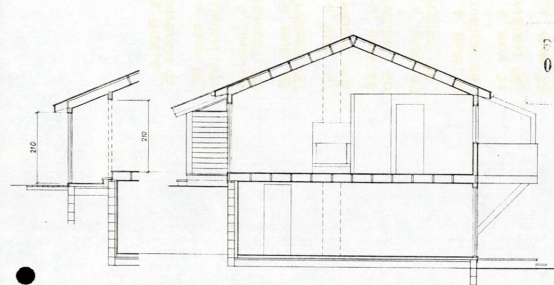
SNITT VINDFANG
