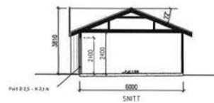
SNITT
