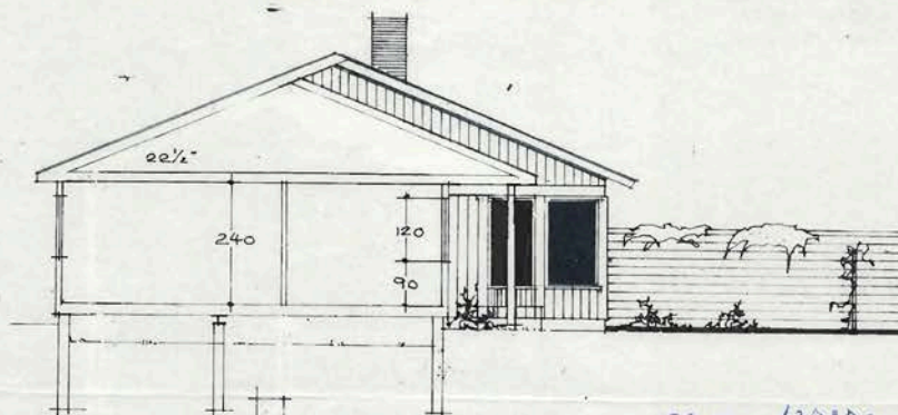
SNITT
