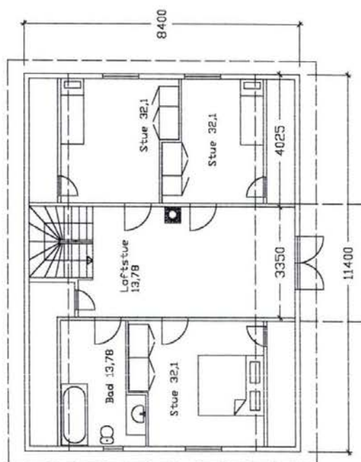
PLANTEGNING 2 ETG.
