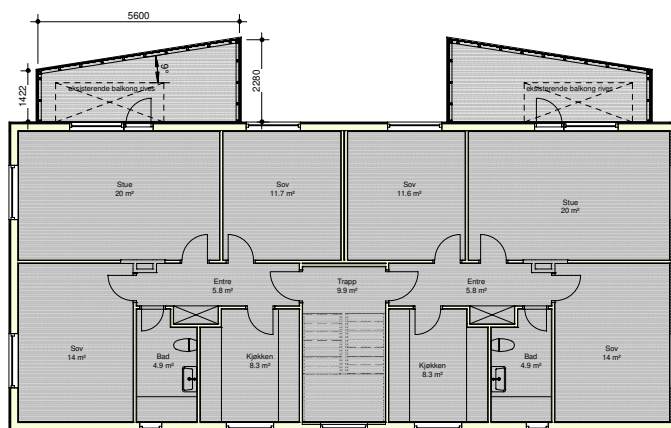
Et. 2 1:100
