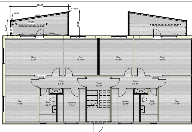
Et. 1 1:100
