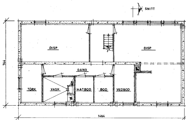
KJELLERPLAN
