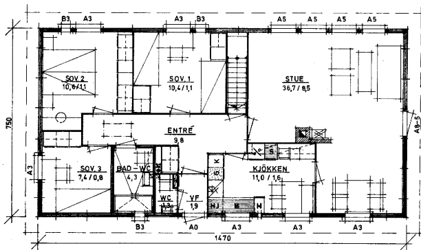
PLAN 1. ETG.
