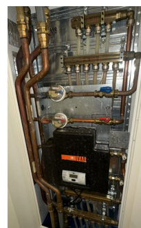
Samleskap med rørkurser og stoppekraner
